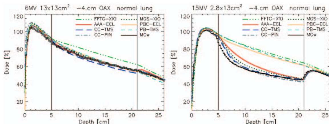
Figura 2. Curve di dose in profondità per il campo 13 \times 13 \text{ cm}^2 , 4 cm fuori dall'asse nel lato della disomogeneità, esperimento normal lung
