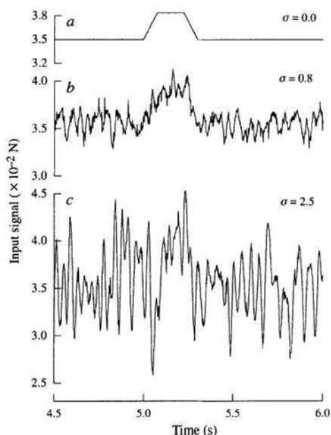
Fig. 5: segnale sottosoglia senza l'aggiunta di rumore (a) e con due livelli di rumore associato (b,c)
